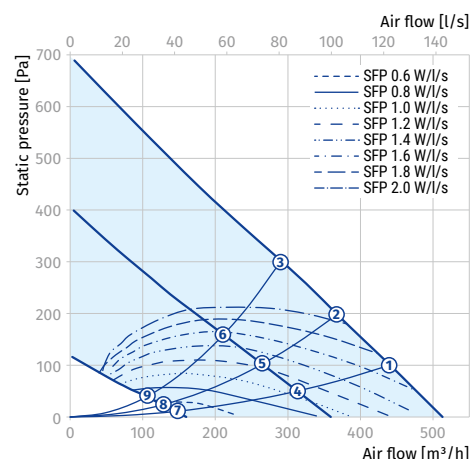
KOMFORT Roto EC D 351
