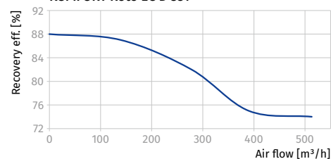
KOMFORT Roto EC D 351-E
