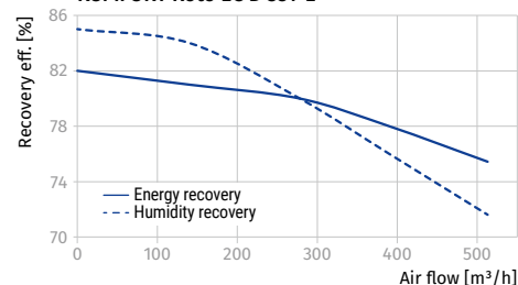
KOMFORT Roto EC D 351-E
